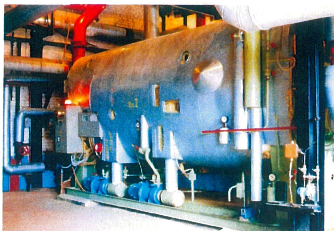
Холодильная установка мощностью 4500 кВт. ОАО «Уфимский нефтеперерабатывающий завод»
