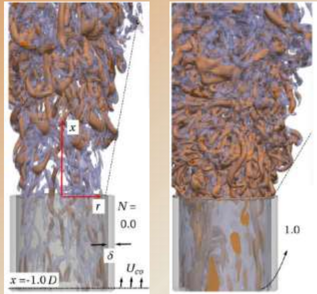
Визуализация вихревых структур при численном моделировании струи, истекающей из вращающейся трубы
